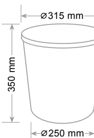
Dimensione-Size-Dimension
