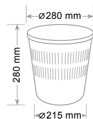
Dimensione-Size-Dimension
